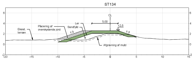
SNIT B-B, 1:150
