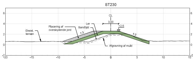
SNIT C-C, 1:150
