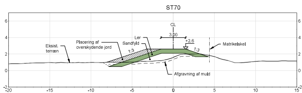
SNIT A-A, 1:150
