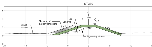
SNIT D-D, 1:150
